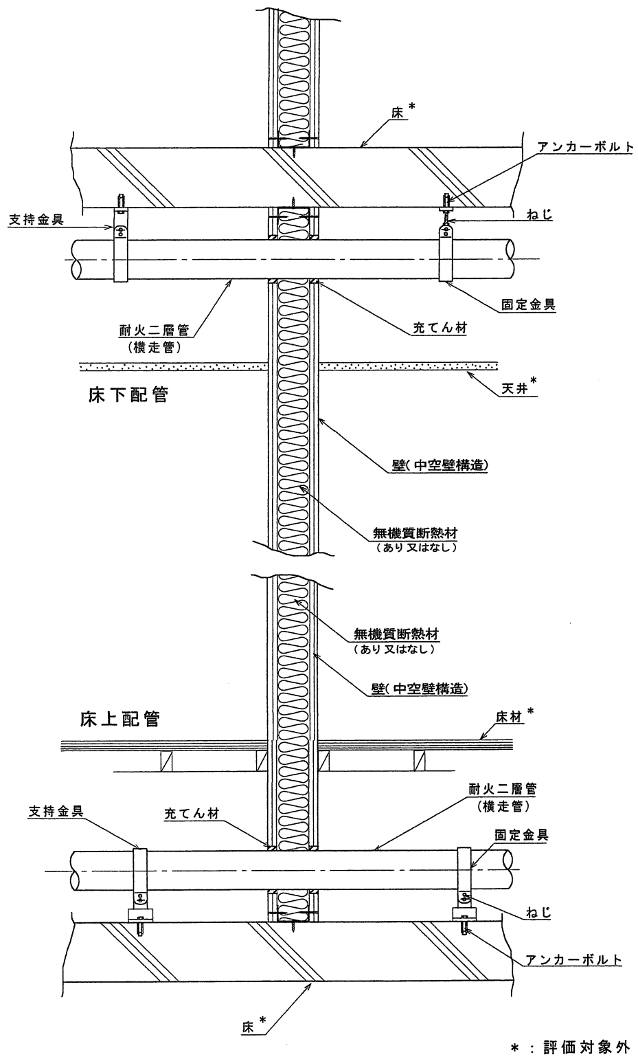
配管施工仕様(1)
