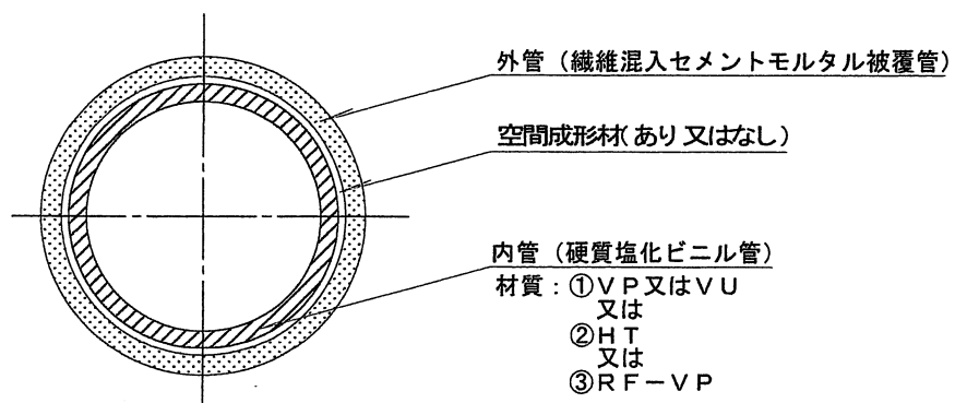
断面詳細図
