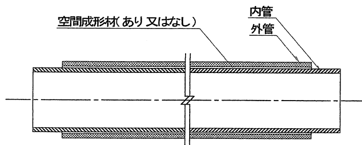
耐火二層管
