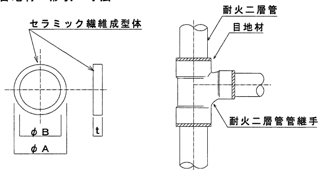
目地材：形状・寸法
